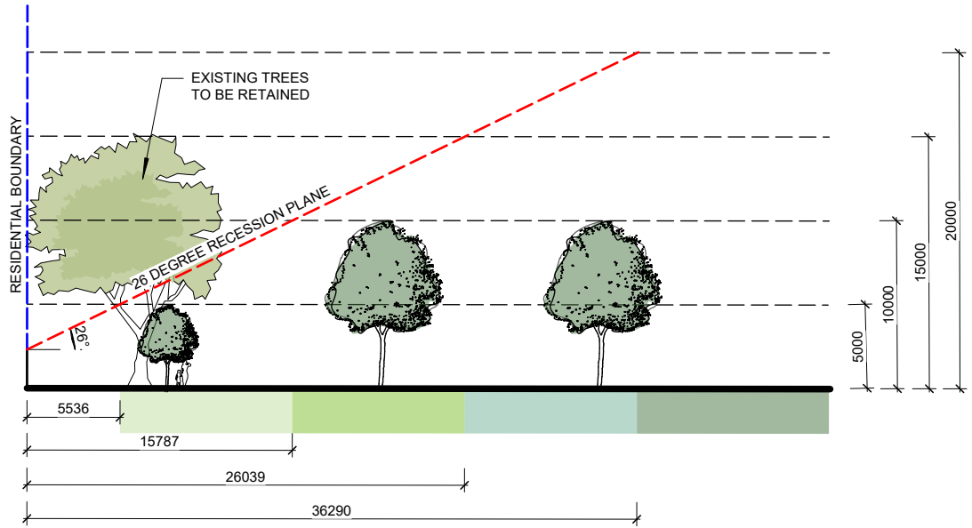
C Section C-C Scale: 1:400
