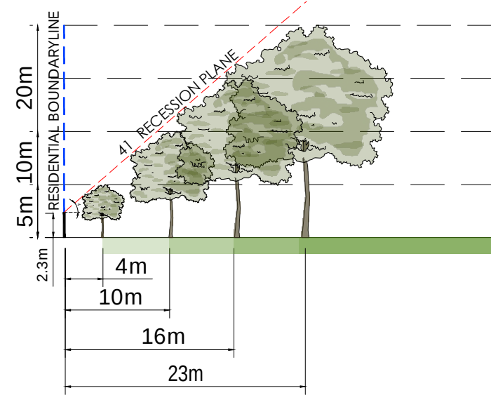
CROSS SECTION DD
